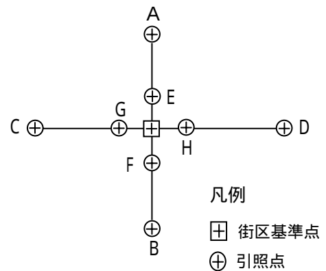
図 3 - 1 - 2 X 型 (E,F,G,H は補助引照点)
